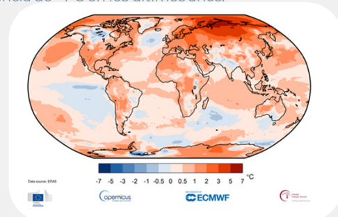
Anomalía de temperatura del aire a 2 metros en 2020, respecto al promedio de 1981-2020.
