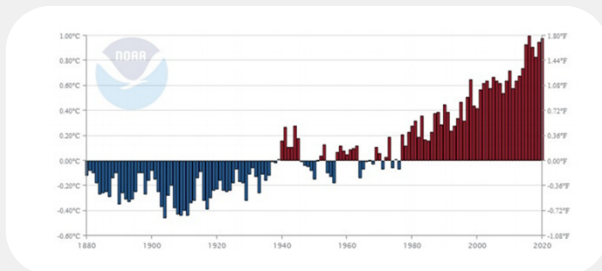
Anomalía de temperatura global de enero a diciembre en el período 1880 - 2020.
